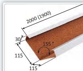
MT Úžlab. úzke, zapus. dlhé Rozvinutá šírka: 0,34 m Potreba: 0,526 ks/m, 1,9 m/ks Hmotnosť: 3 kg/ks Číslo dielu: D 04050210
