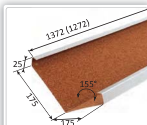
MT Úžlab. šir. zapustené, krátke Rozvinutá šírka: 0,456 m Potreba: 0,786 ks/m, 1,272 m/ks Hmotnosť: 2,8 kg/ks Číslo dielu: D 04050320
