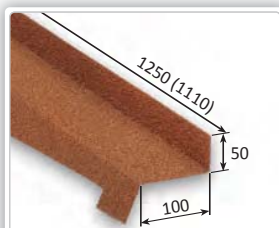
MT Ukončovacia lišta k murivu pravá Rozvinutá šírka: - Potreba: 0,9 ks/m, 1,11 m/ks Hmotnosť: 1,2 kg/ks Číslo dielu: D 04030400
