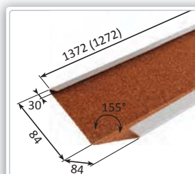
MT Úžlab. úzke, nezapus. krátke Rozvinutá šírka: 0,228 m Potreba: 0,786 ks/m, 1,272 m/ks Hmotnosť: 1,4 kg/ks Číslo dielu: D 04050520
