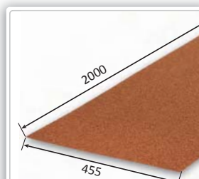
MT Rovný plech 2000x455 Rozvinutá šírka: 0,455 m Potreba: - Hmotnosť: 4,3 kg/ks Číslo dielu: D 04060100
