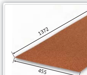
MT Rovný plech 1372x455 Rozvinutá šírka: 0,455 m Potreba: - Hmotnosť: 2,9 kg/ks Číslo dielu: D 04060200
