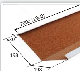
MT Úžlab. šir. nezapus. dlhé Rozvinutá šírka: 0,456 m Potreba: 0,526 ks/m, 1,9 m/ks Hmotnosť: 4 kg/ks Číslo dielu: D 04050810
