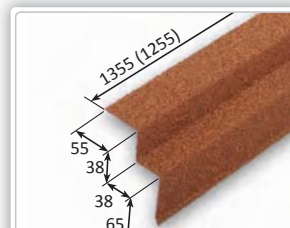
MT Odkvap. lišta pod kryt. úzka Rozvinutá šírka: 0,200 m Potreba: 0,8 ks/m, 1,255 m/ks Hmotnosť: 1,3 kg/ks Číslo dielu: D 04040130
