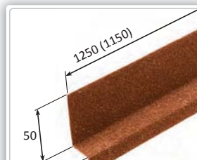
MT Nos okrajovej lišty Rozvinutá šírka: 0,110 m Potreba: 0,869 ks/m, 1,15 m/ks Hmotnosť: 0,7 kg/ks Číslo dielu: D 04030514
