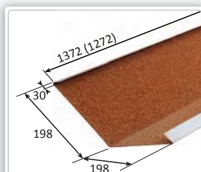
MT Úžlab. šir. nezapus. krátke Rozvinutá šírka: 0,456 m Potreba: 0,786 ks/m, 1,272 m/ks Hmotnosť: 2,8 kg/ks Číslo dielu: D 04050720
