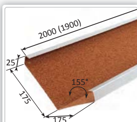
MT Úžlab. šir. zapustené, dlhé Rozvinutá šírka: 0,456 m Potreba: 0,526 ks/m, 1,9 m/ks Hmotnosť: 4 kg/ks Číslo dielu: D 04050410
