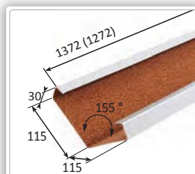
MT Úžlab. úzke, zapus. krátke Rozvinutá šírka: 0,34 m Potreba: 0,786 ks/m, 1,272 m/ks Hmotnosť: 2 kg/ks Číslo dielu: D 04050120
