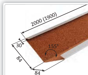
MT Úžlab. úzke, nezapus. dlhé Rozvinutá šírka: 0,228 m Potreba: 0,526 ks/m, 1,9 m/ks Hmotnosť: 2 kg/ks Číslo dielu: D 04050610
