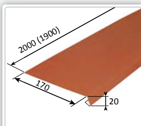
MT Odkvap. lišta pod fóliu Rozvinutá šírka: 0,200 m Potreba: 0,526 ks/m, 1,9 m/ks Hmotnosť: 1,7 kg/ks Číslo dielu: D 04040414 (3)
