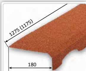
MRo Lemovanie pod hrebenáč Rozvinutá šírka: - Potreba: 0,851 ks/m, 1,9 m/ks Hmotnosť: 1,64 kg/ks Číslo dielu: D 04070100
