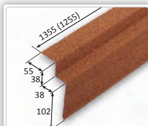
MT Odkvap. lišta pod kryt. široká Rozvinutá šírka: 0,235 m Potreba: 0,8 ks/m, 1,255 m/ks Hmotnosť: 1,6 kg/ks Číslo dielu: D 04040230
