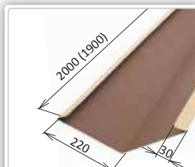
MŠt410 Úžľabie široké, nezap. Rozvinutá šírka: 0,500 m Potreba: 0,526 ks/m, 1,9 m/ks Hmotnosť: 4 kg/ks Číslo dielu: D 03050820
