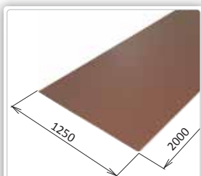
MŠt Rov. pl. 1250x2000 mm Rozvinutá šírka: 1,250 m Potreba: - Hmotnosť: 10 kg/ks Číslo dielu: D 03060120
