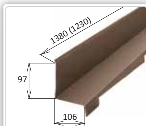
MŠt410 Ukončovacia lišta ľavá Rozvinutá šírka: - Potreba: 0,81 ks/m, 1,23 m/ks Hmotnosť: 1,28 kg/ks Číslo dielu: D 03030700
