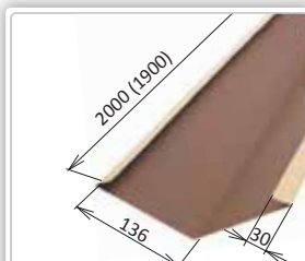
MŠt410 Úžľabie úzke, nezap. Rozvinutá šírka: 0,333 m Potreba: 0,526 ks/m, 1,9 m/ks Hmotnosť: 2,6 kg/ks Číslo dielu: D 03050720
