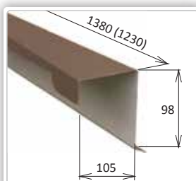
MŠt410 Okrajová lišta pravá Rozvinutá šírka: - Potreba: 0,81 ks/m, 1,23 m/ks Hmotnosť: 1,28 kg/ks Číslo dielu: D 03030400
