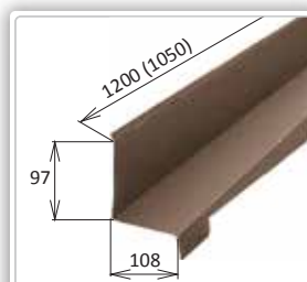
MŠt350 Ukončovacia lišta ľavá Rozvinutá šírka: - Potreba: 0,95 ks/m, 1,05 m/ks Hmotnosť: 1,1 kg/ks Číslo dielu: D 03030500
