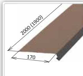
MŠt410 Odkvap. lišta pod fóliu Rozvinutá šírka: 0,200 m Potreba: 0,526 ks/m, 1,9 m/ks Hmotnosť: 1,6 kg Číslo dielu: D 03040220
