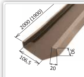
MŠt 350 Úžľabie úzke, zap. Rozvinutá šírka: 0,313 m Potreba: 0,526 ks/m, 1,9 m/ks Hmotnosť: 2,5 kg/ks Číslo dielu: D 03050110
