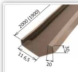
MŠt 410 Úžľabie úzke, zap. Rozvinutá šírka: 0,333 m Potreba: 0,526 ks/m, 1,9 m/ks Hmotnosť: 2,6 kg/ks Číslo dielu: D 03050520
