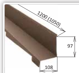
MŠt350 Ukončovacia lišta pravá Rozvinutá šírka: - Potreba: 0,95 ks/m, 1,05 m/ks Hmotnosť: 1,1 kg/ks Číslo dielu: D 03030600
