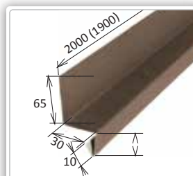
MŠt Nos okrajovej lišty Rozvinutá šírka: 0,125 m Potreba: 0,526 ks/m, 1,9 m/ks Hmotnosť: 1 kg/ks Číslo dielu: D 03030900
