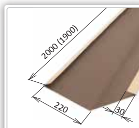
MŠt 350 Úžľabie široké, nezap. Rozvinutá šírka: 0,500 m Potreba: 0,526 ks/m, 1,9 m/ks Hmotnosť: 4 kg/ks Číslo dielu: D 03050410
