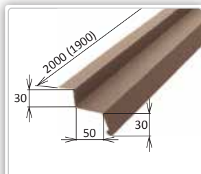
MŠt410 Odkvap. lišta pod krytinu Rozvinutá šírka: 0,167 m Potreba: 0,526 ks/m, 1,9 m/ks Hmotnosť: 1,3 kg/ks Číslo dielu: D 03040120
