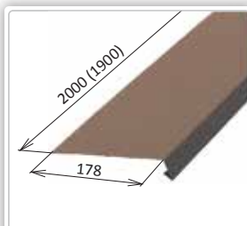
MŠt350 Odkvap. lišta pod fóliu Rozvinutá šírka: 0,208 m Potreba: 0,526 ks/m, 1,9 m/ks Hmotnosť: 1,6 kg/ks Číslo dielu: D 03040210
