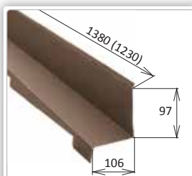
MŠt410 Ukončovacia lišta pravá Rozvinutá šírka: - Potreba: 0,81 ks/m, 1,23 m/ks Hmotnosť: 1,28 kg/ks Číslo dielu: D 03030800
