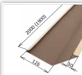
MŠt 350 Úžľabie úzke, nezap. Rozvinutá šírka: 0,313 m Potreba: 0,526 ks/m, 1,9 m/ks Hmotnosť: 2,5 kg/ks Číslo dielu: D 03050310
