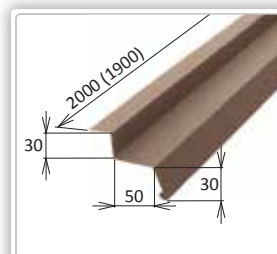
MŠt350 Odkvap. lišta pod krytinu Rozvinutá šírka: 0,156 m Potreba: 0,526 ks/m, 1,9 m/ks Hmotnosť: 1,25 kg/ks Číslo dielu: D 03040110
