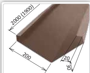
MKp 410 Úžľabie široké, zap. Rozvinutá šírka: 0,500 m Potreba: 0,526 ks/m, 1,9 m/ks Hmotnosť: 4,0 kg/ks Číslo dielu: D 03050620
