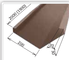
MŠt 350 Úžľabie široké, zap. Rozvinutá šírka: 0,500 m Potreba: 0,526 ks/m, 1,9 m/ks Hmotnosť: 4,0 kg/ks Číslo dielu: D 03050210
