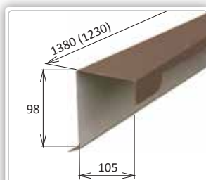
MŠt410 Okrajová lišta ľavá Rozvinutá šírka: - Potreba: 0,81 ks/m, 1,23 m/ks Hmotnosť: 1,28 kg/ks Číslo dielu: D 03030300
